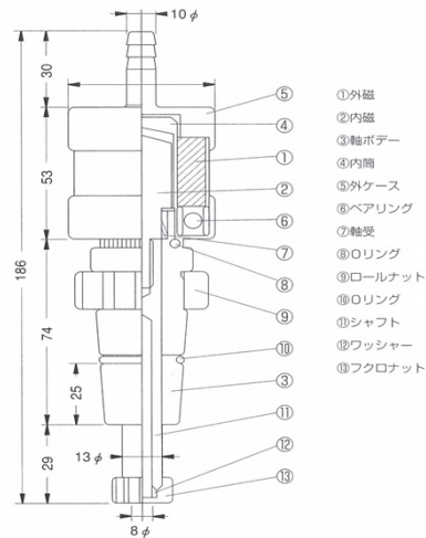
1005部品図
